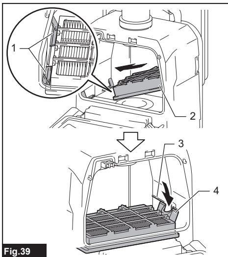
► 1. Soporte 2. Filtro HEPA 3. Nervadura 4. Solapa
