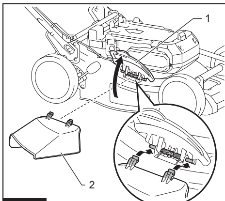
► 1. Cubierta del lado derecho 2. Accesorio de descarga
